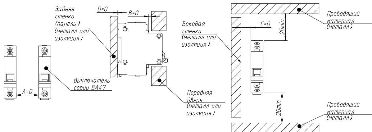
Рисунок 8 — Периметр безопасности
