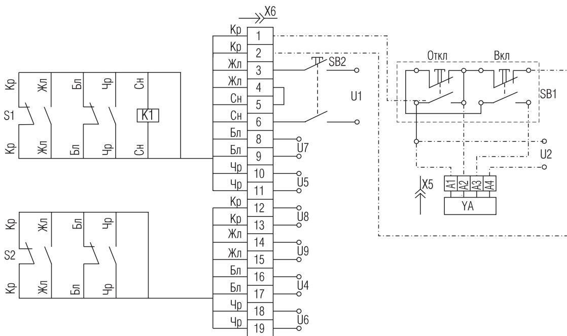
Рисунок В.6.1. Схема электрическая соединений дополнительных сборочных единиц выключателей выдвигного исполнения (ручной или электромагнитный привод, вспомогательные, дополнительные вспомогательные контакты)
