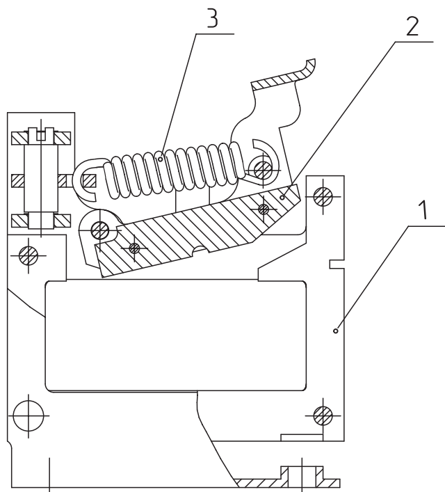
Рисунок 2. Электромагнитный расцепитель
